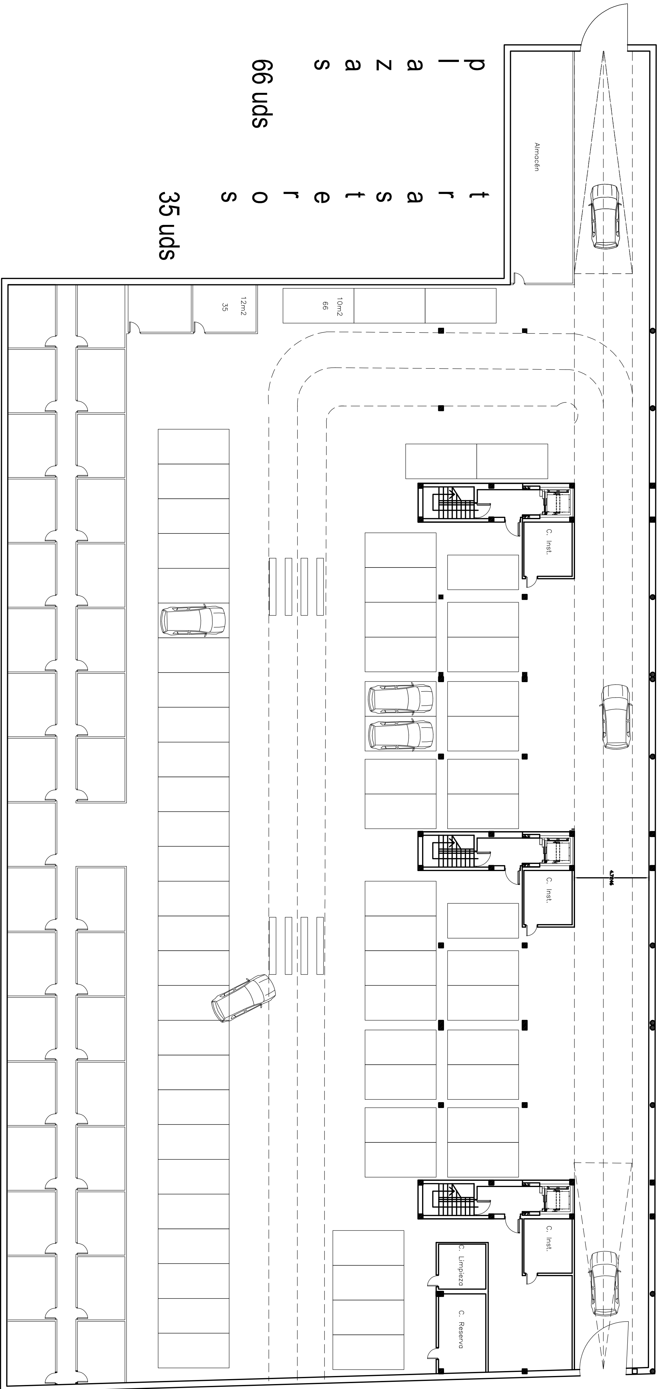
PLANTA GARAJES C. -1.00 E. 1150 Diseño de Vivienda, Cuenca
